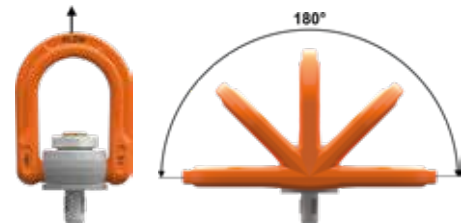
Bild 1: erlaubte Belastungsrichtungen die bei bestimmungsgemäßem Gebrauch auftreten können.
