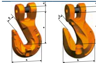
Form mit Stützsattel
