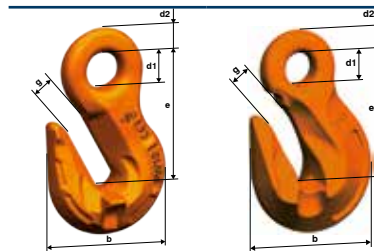
Forme avec selle d'appui
