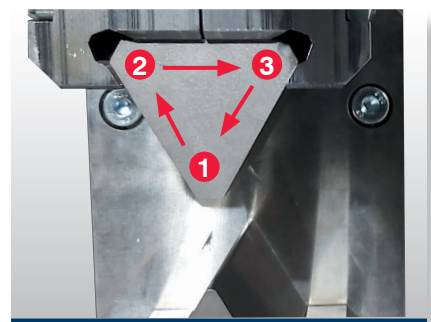
Klingen wendbar (wiederverwendbar)
