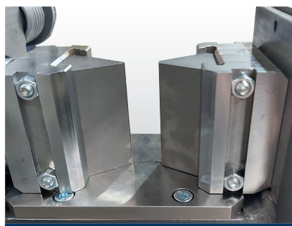
Schneidbereich mit Hartmetallmesser und Messerführung
